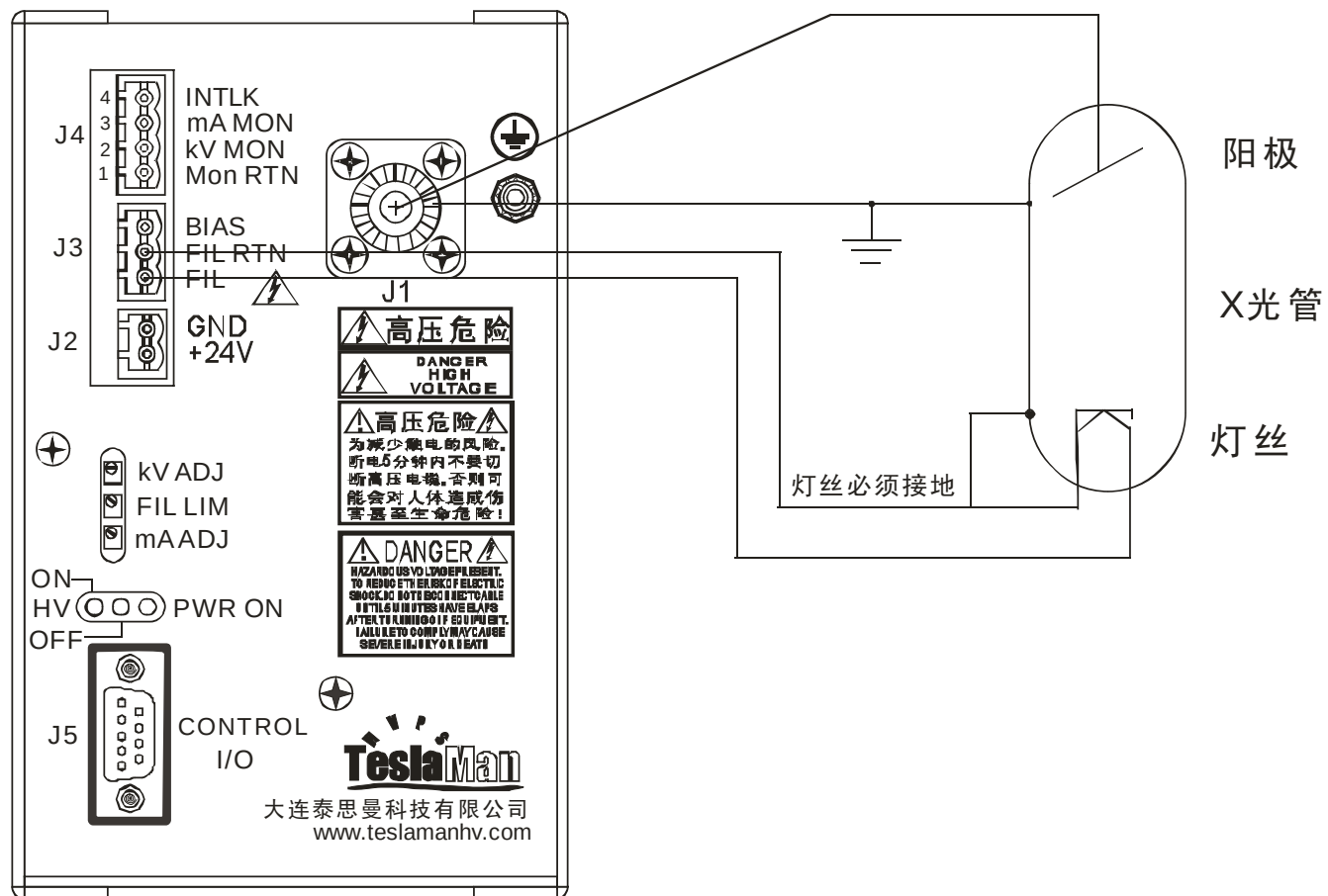
图 3.1 典型工作接线图
